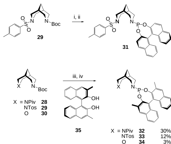
Scheme 11. Synthesis of phosphoramidites 31–34 : i) TFA, CH 2 Cl 2 , 30 min, RT; ii) ClP(BINOL), 10a , Et 3 N, toluene, 12 h, RT, 51 %; iii) TFA, CH 2 Cl 2 , 30 min, RT; iv) PCl 3 , Et 3 N, THF, 1 h, 0 °C, then 35 , Et 3 N, THF, 12 h, RT.
