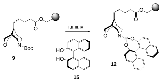
Scheme 5. Alternative synthesis of phosphoramidite 12 : i) TFA, CH 2 Cl 2 , 30 min; ii) Et 3 N, CH 2 Cl 2 , 15 min; iii) PCl 3 , Et 3 N, THF, 1 h; iv) 15 , Et 3 N, THF, 12 h.
